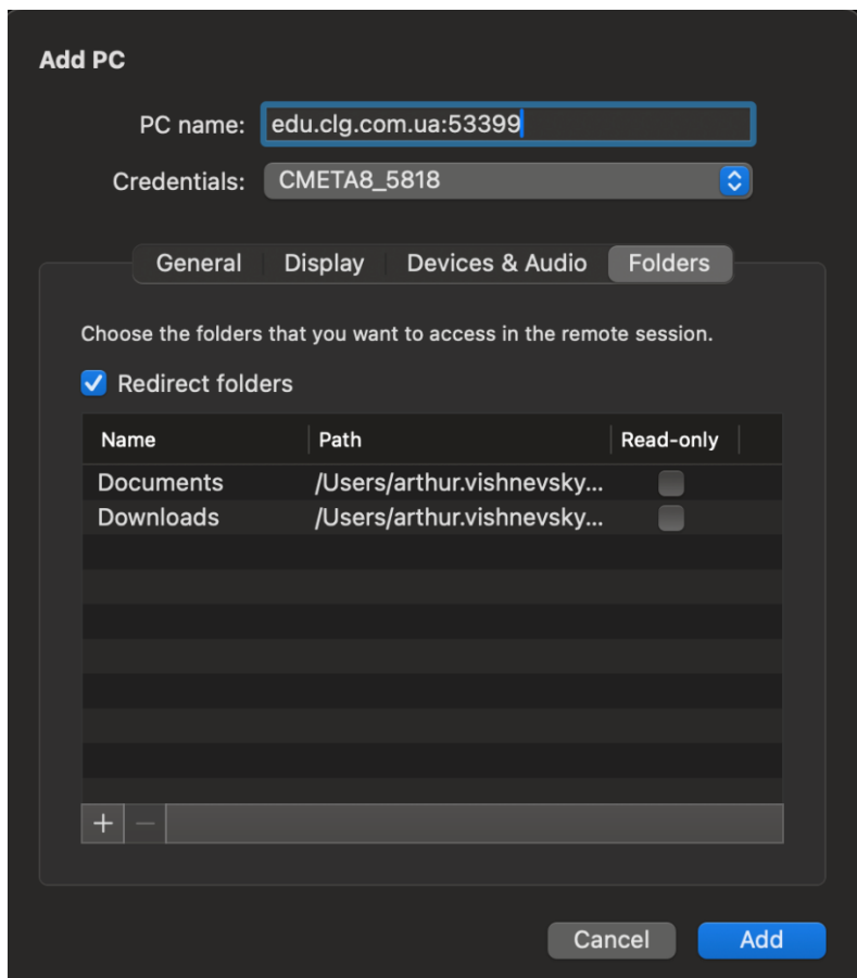
Рис. 8. Папки "Documents" та "Download" підключені до відділеного робочого столу
